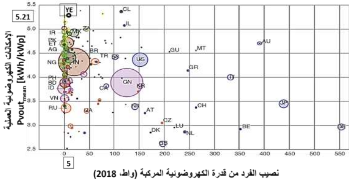
الشكل (15) يبين إمكانيات العملية مقارنة بالسعة الكهروضوئية المركبة للشخص في 2018.
