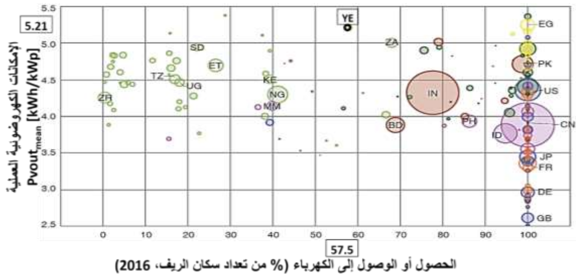
الشكل (17) يبين إمكانيات الطاقة الكهروضوئية العملية مقابل حصول سكان الريف على الكهرباء
