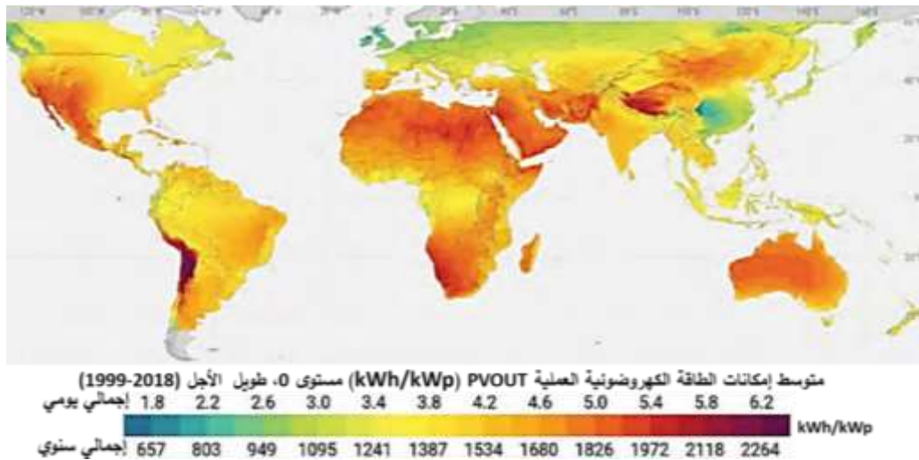
الشكل (6) يبين توزيع متوسط الإمكانات الكهروضوئية العملية على المدى الطويل (المستوى 0)
